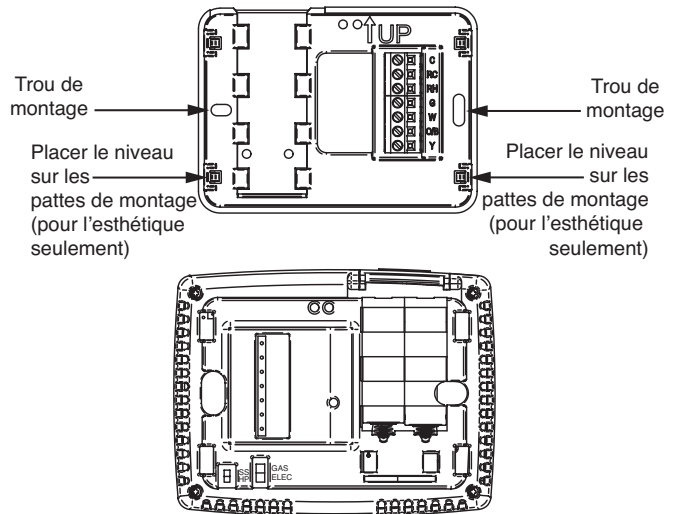
Figure 2. Socle du thermostat et vue de l'arrière du thermostat
